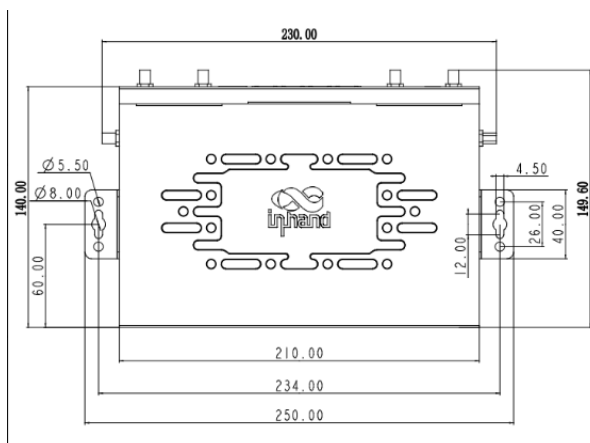
正视图
