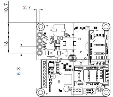
BOT层
