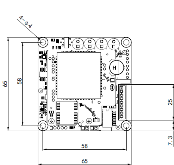
TOP层
