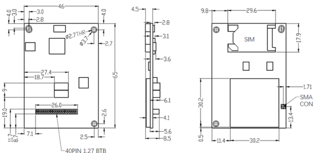
InDTU323L 的尺寸
